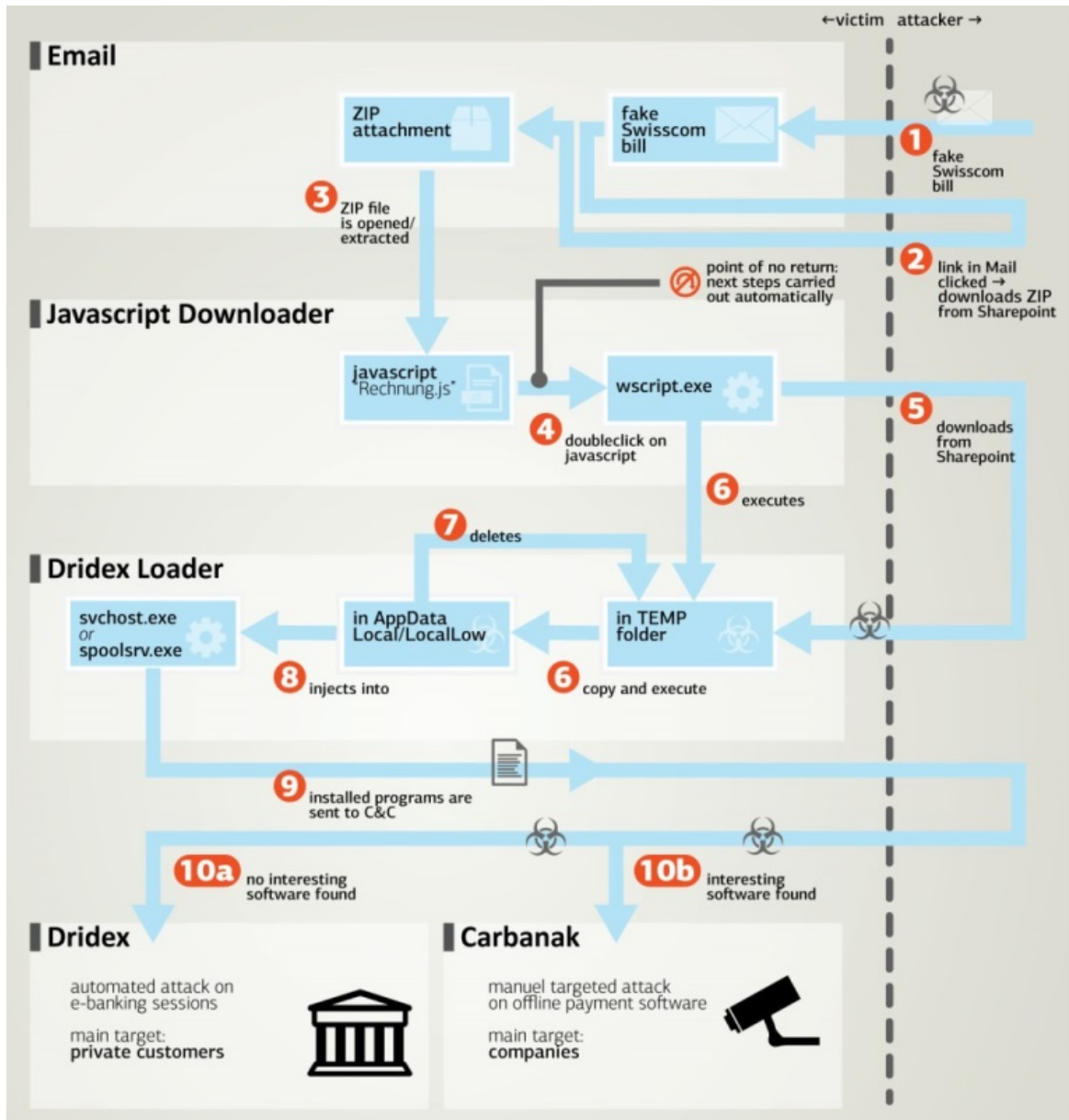
Fig. 4: Schéma du mode d'infection à l'œuvre pendant la vague de pourriels de février 2017 reposant sur de fausses factures Swisscom.
